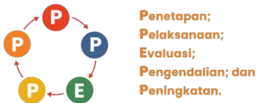
Gambar 1. Siklus PPEPP
